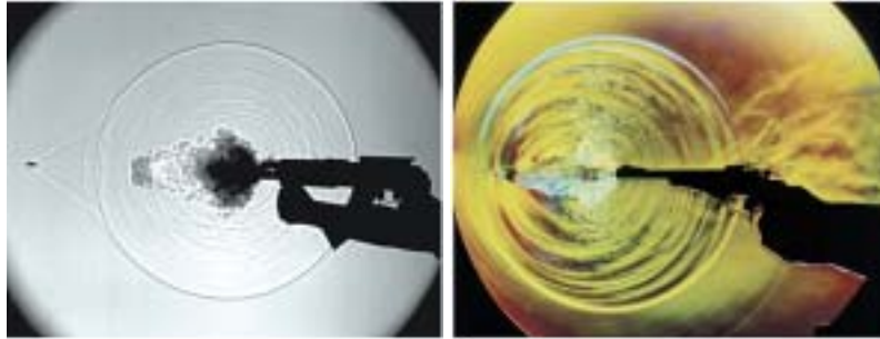
На рисунке слева — начало очереди из автомата с глушителем. Темно-синее облачко — невидимые глазу пороховые газы. Справа — выстрел из пистолета. На приборе отчетливо видны кольца звуковых волн.
